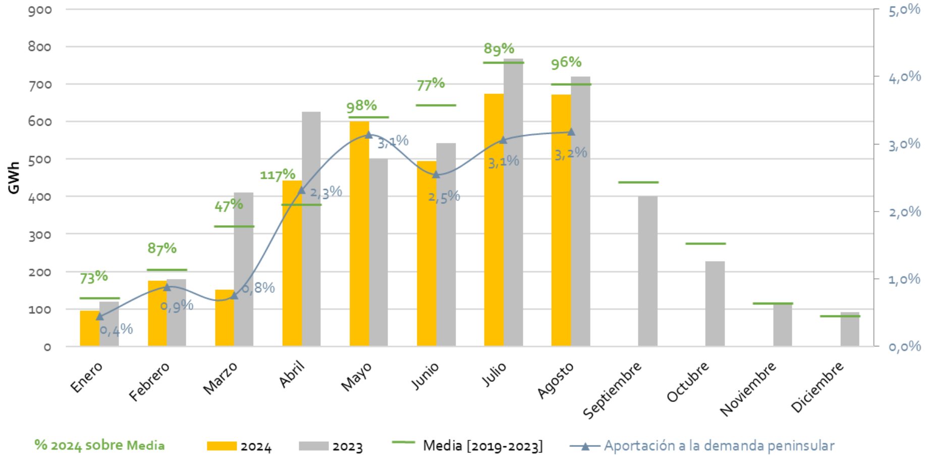
Termosolar Comparativa de generación mensual
