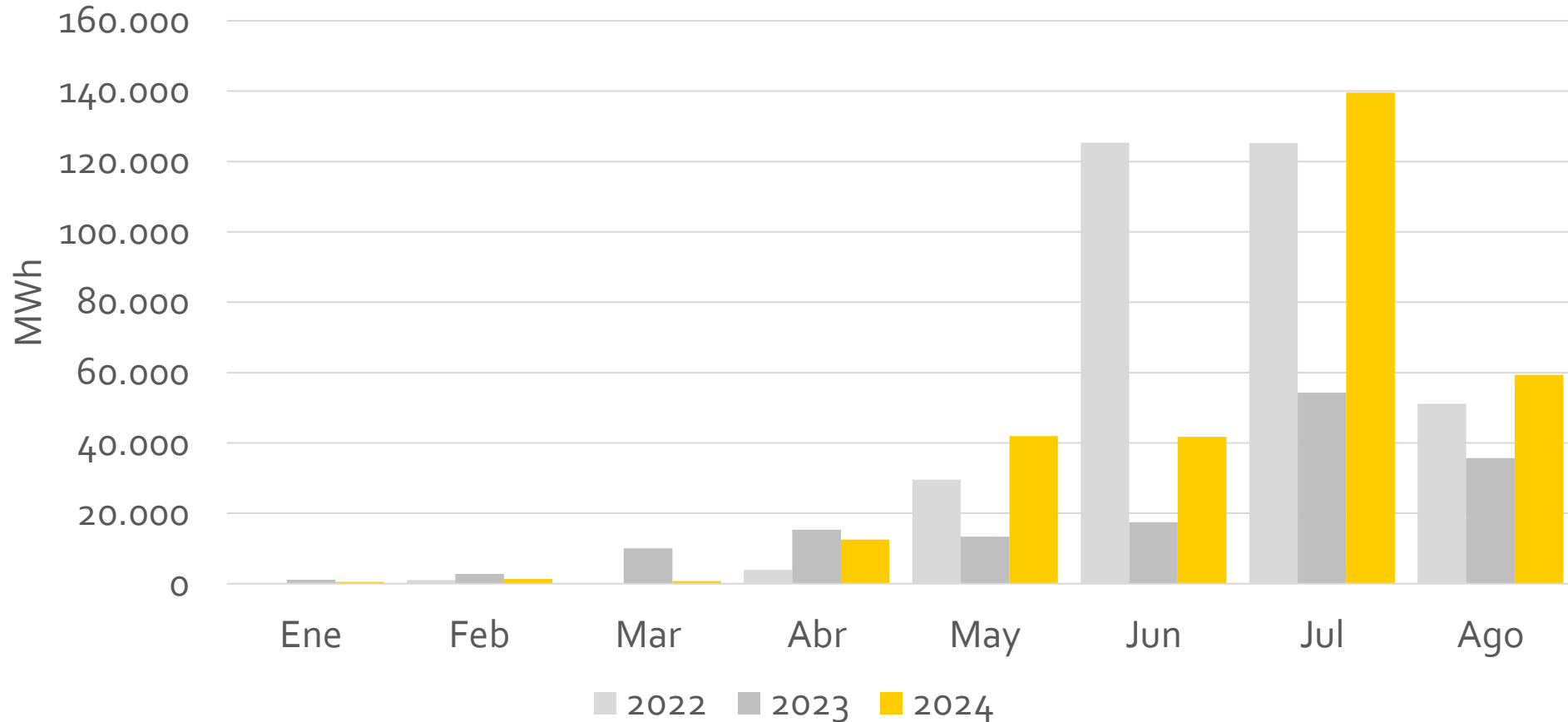
Restricciones Técnicas mensuales CSP (MWh)
