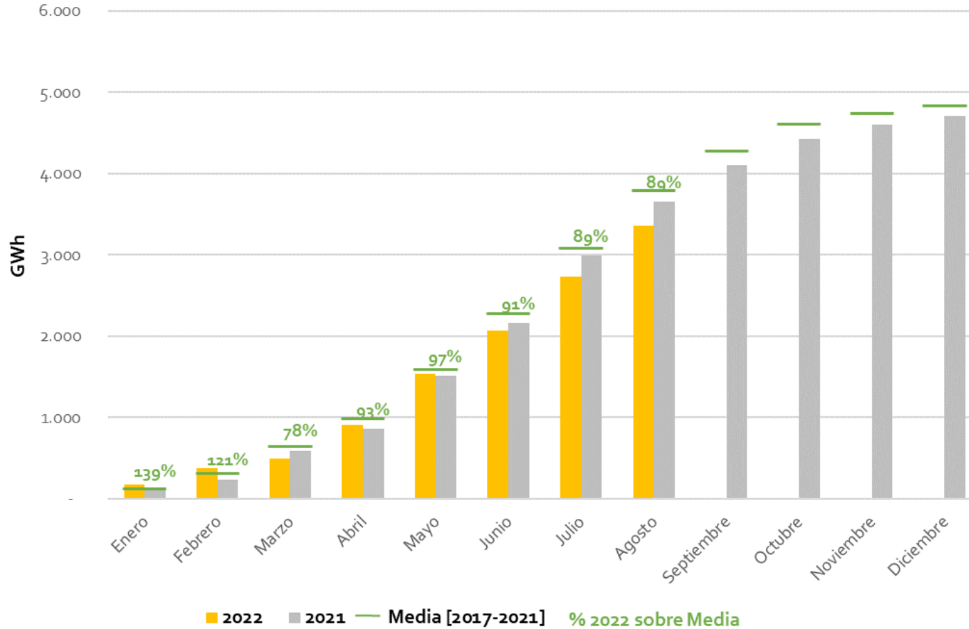
Solar Termoeléctrica Generación Medida Acumulada
