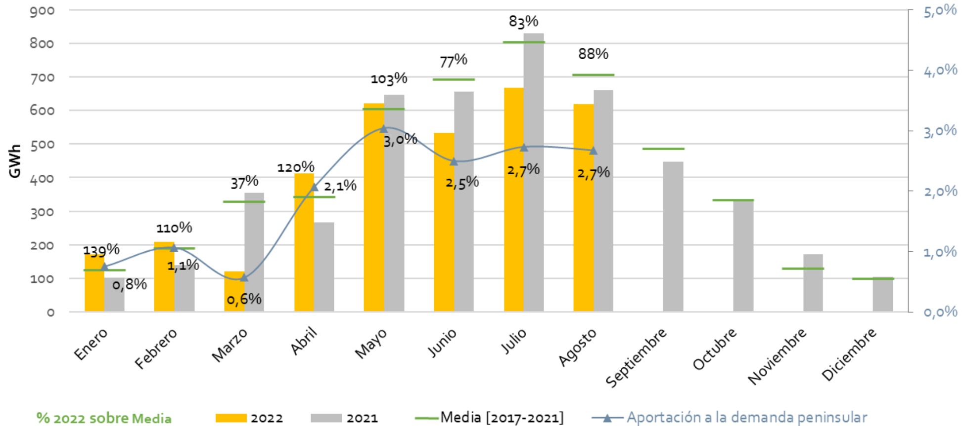
Solar Térmoelectrica Comparativa de generación mensual
